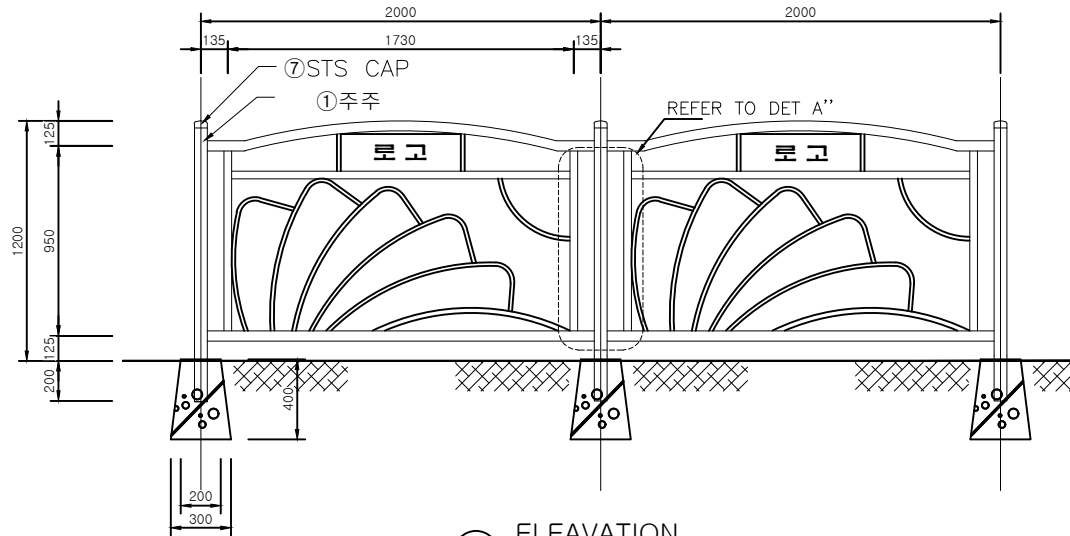
ELEVATION SCALE:NONE
