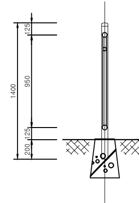
SIDE VIEW SCALE:NONE
