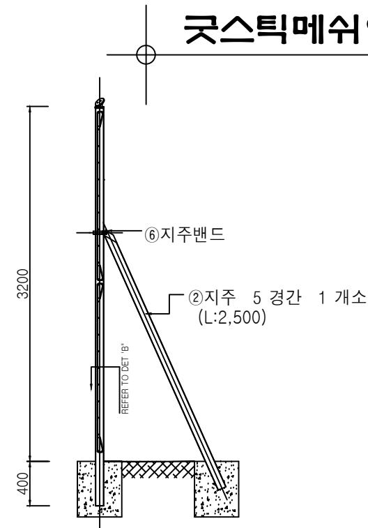
SIDE VIEW SCALE: NONE
