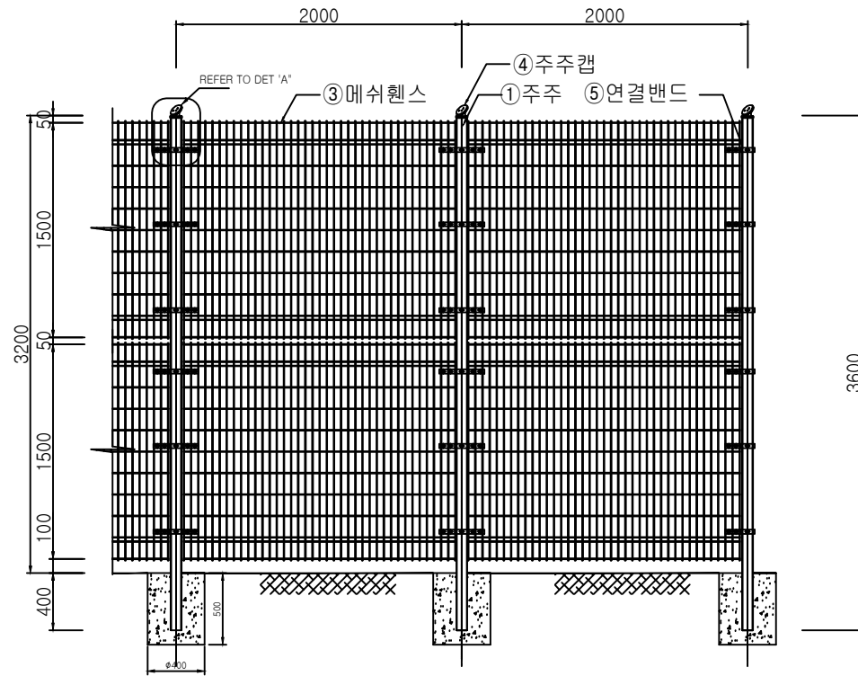
ELEVATION SCALE: NONE
