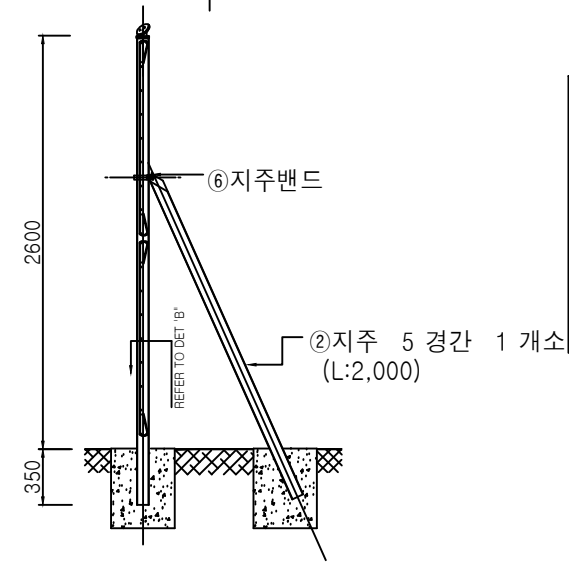
SIDE VIEW SCALE: NONE
