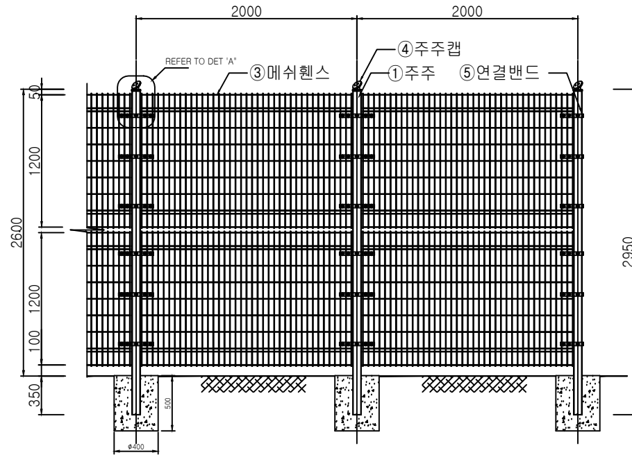
ELEVATION SCALE: NONE
