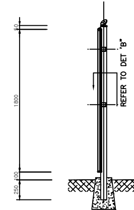
SIDE VIEW SCALE: NONE
