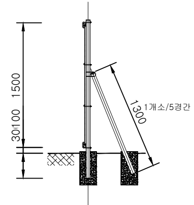
SIDE VIEW SCALE:NONE
