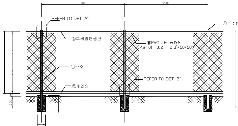
ELEVATION SCALE:NONE
